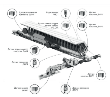
Современность. Система радиомониторинга комплекса и очистного комбайна.
